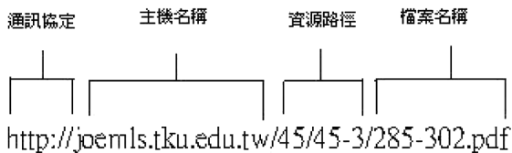
圖1 URLs範例
